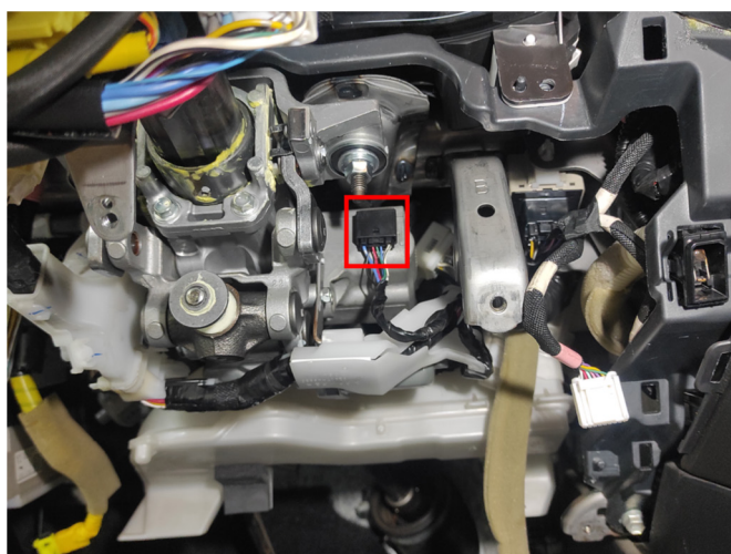
Место подключения разблокировки руля
