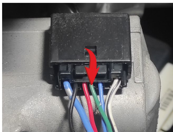
Разблокировка руля (зеленый провод)
