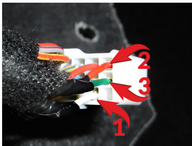
Подключение к цепям запуска двигателя: 1 – АСС (белый провод); 2 – Зажигание 1 (красный провод); 3 – Стартер (зеленый провод).
