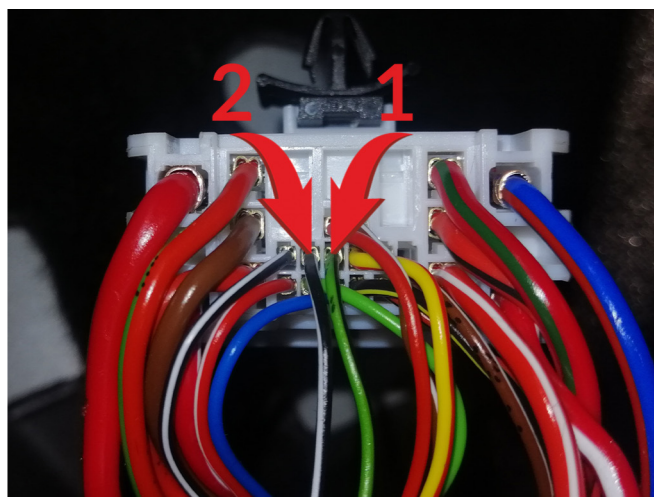
Подключение к цепям запуска двигателя: 1 – Зажигание 1 (зеленый/черный, контакт №14); 2 – Зажигание 2 (черный/белый, контакт №13)
