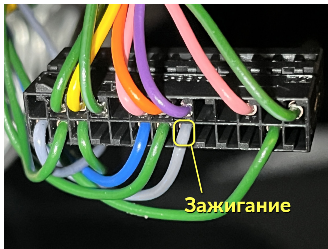
Подключение к цепям запуска двигателя: Зажигание – серый провод, контакт № 34 «+»
