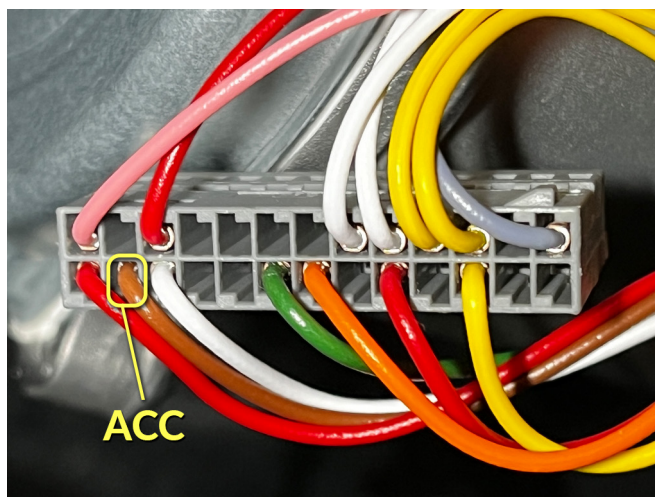
Подключение к цепям запуска двигателя: Аксессуары – коричневый провод, контакт № 25 «+»
