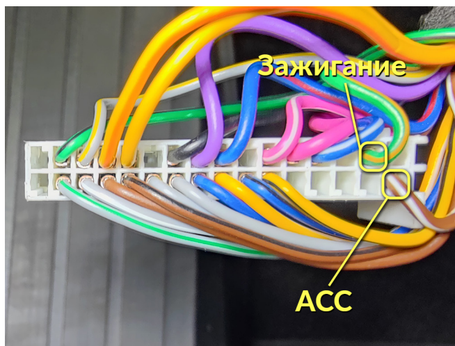
Подключение к цепям запуска двигателя: ACC – коричнево-белый провод, контакт № 32 «+»; Зажигание – зелено-желтый провод, контакт №15 «+».
