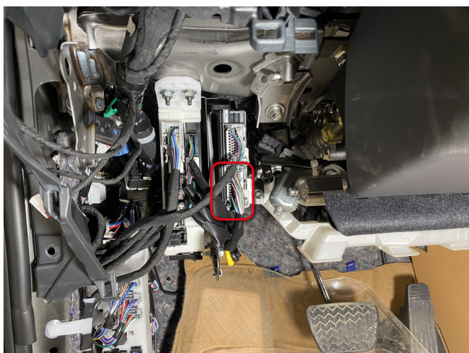
Черный 54 контактный разъем блока Hybrid ECU, слева от рулевой колонки
