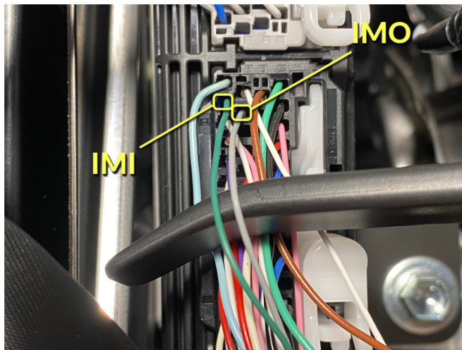
Подключение к шине данных: IMO – серый провод, контакт № 39; IMI – зеленый провод, контакт № 53.
