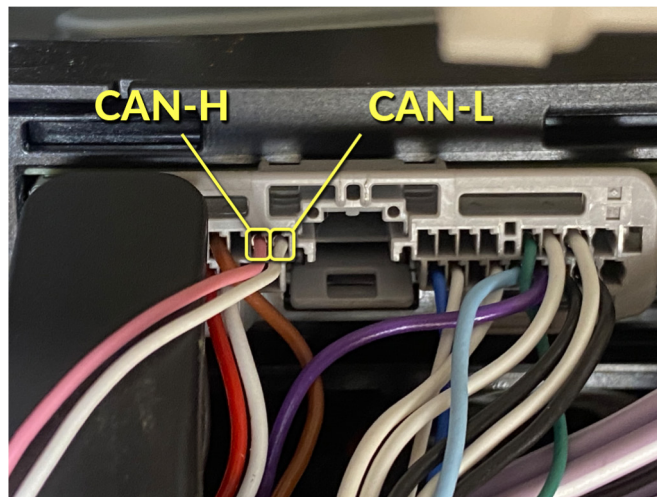
CAN-H - розовый провод, контакт №25; CAN-L - белый провод, контакт №26.
