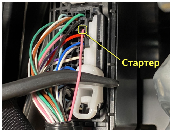
Подключение силовых цепей запуска двигателя: Стартер – розовый провод, контакт № 11 «+»;
